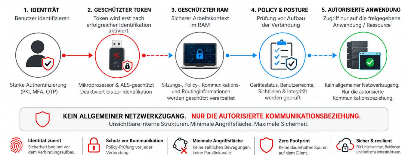
Abb. 2: Fünf Schritte vom identifizierten Benutzer zur autorisierten Anwendung.
